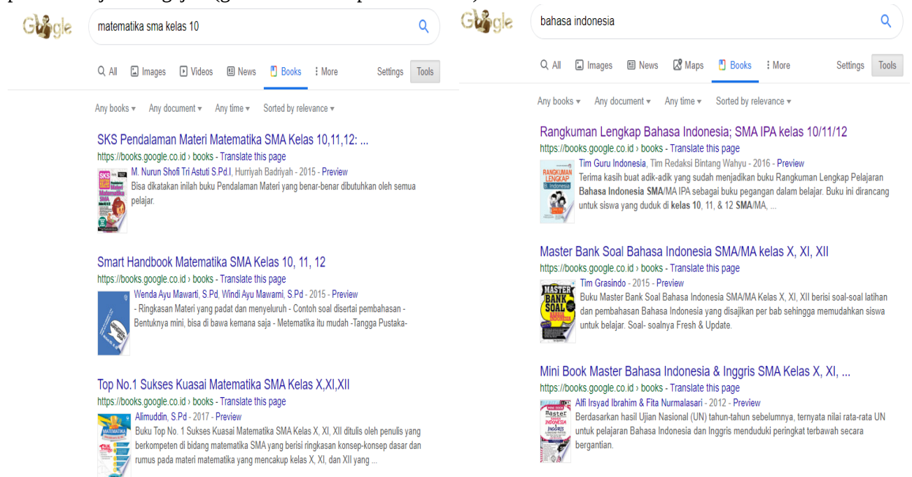
Gambar 3 Mendapatkan E-Book
