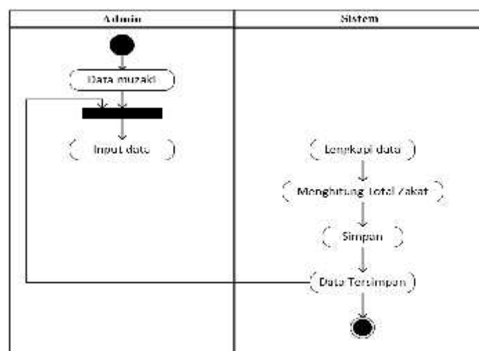
Gambar 3.6 Rancangan Activity Diagram Penerimaan Zakat Fitrah
