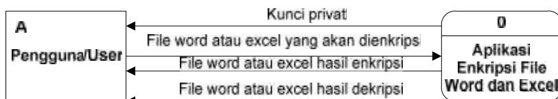
Gambar 5. Diagram konteks
