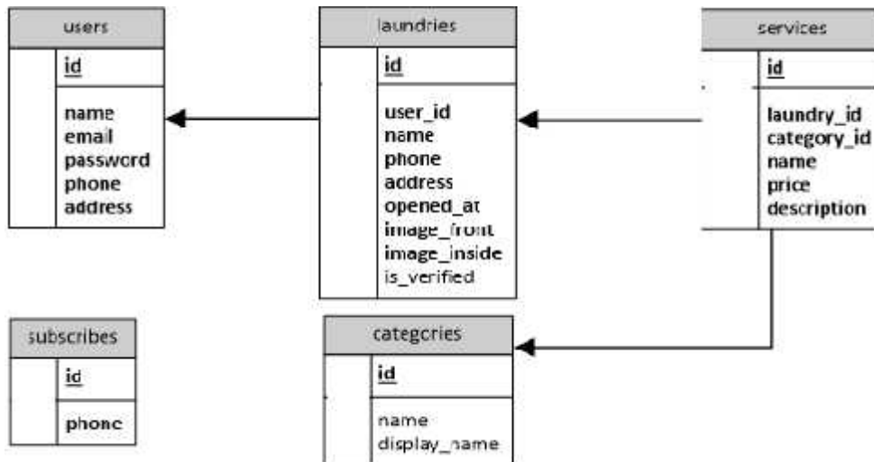
Gambar 5 Rancangan Database
