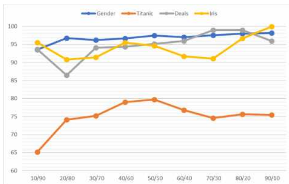
Gambar 5. Nilai Akurasi Dataset Gender, Titanic, Deals, dan Iris pada Sembilan Komposisi Jumlah Data Training dan Data Testing.
