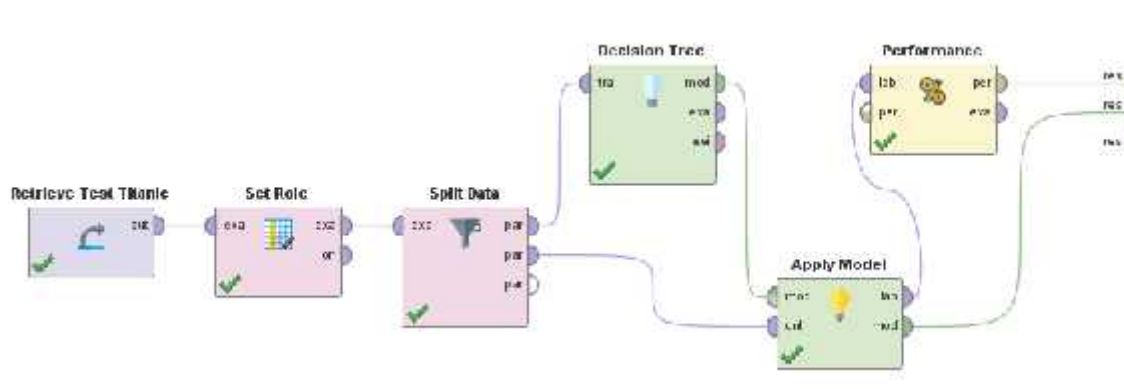
Gambar 2. Workflow Rapid Miner untuk Menguji Akurasi Komposisi Data Training dan Testing.
