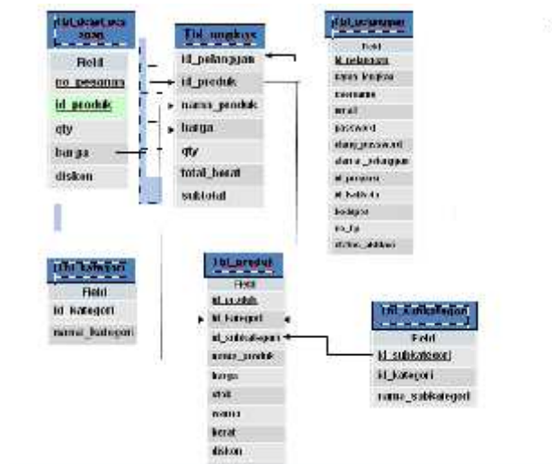
Gambar 6. Relasi Antar Tabel
