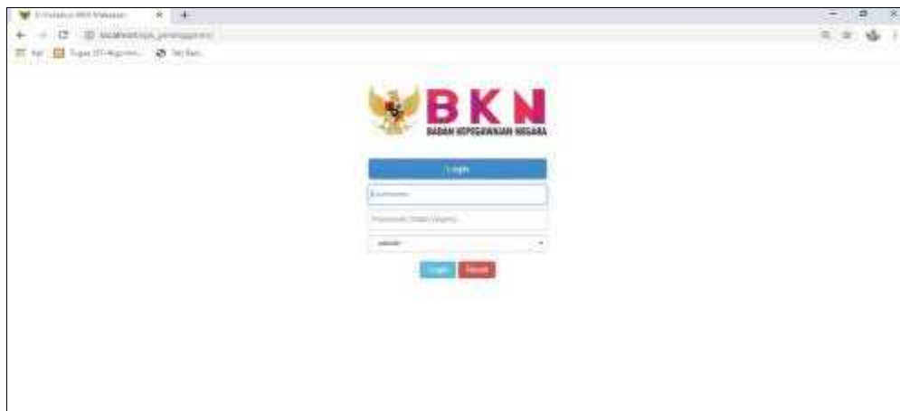
Gambar 1. Tampilan Login
