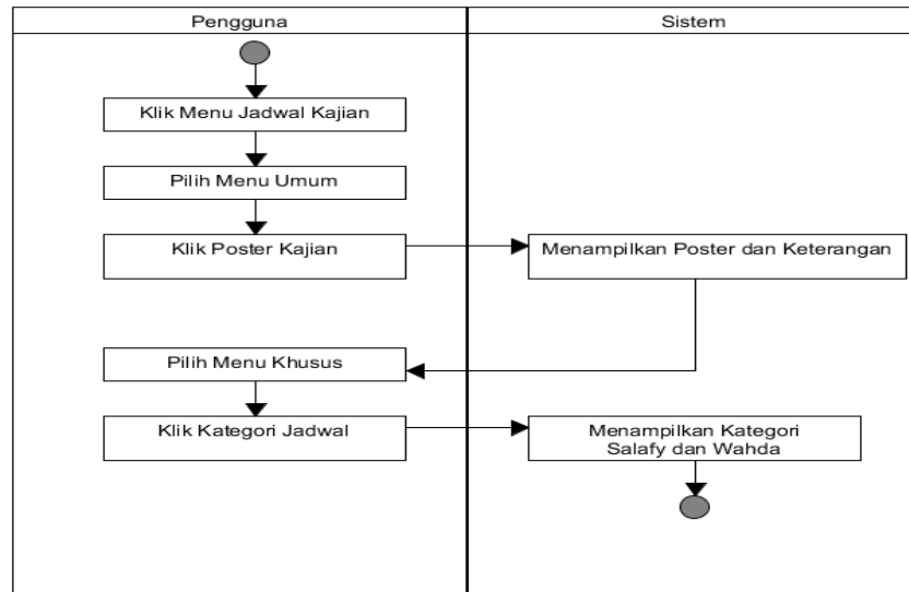
Gambar 3.9 Activity Diagram Input Jadwal Kajian Penyelenggara
