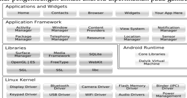
Gambar 2.1 Arsitektur Android
