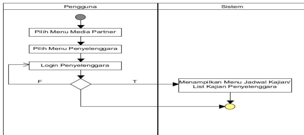
Gambar 3.10 Activity Diagram Jadwal Kajian Penyelenggara
