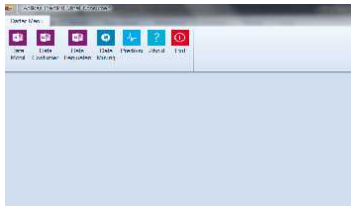
Gambar 7. Menu utama
