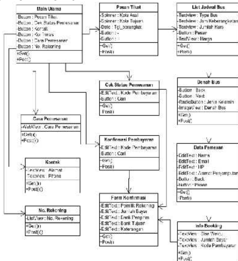
Gambar 2. Class Diagram Sistem Penjualan Tiket Bus
