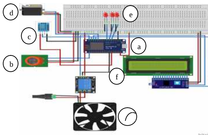
Gambar 4 skema Rancangan Alat
