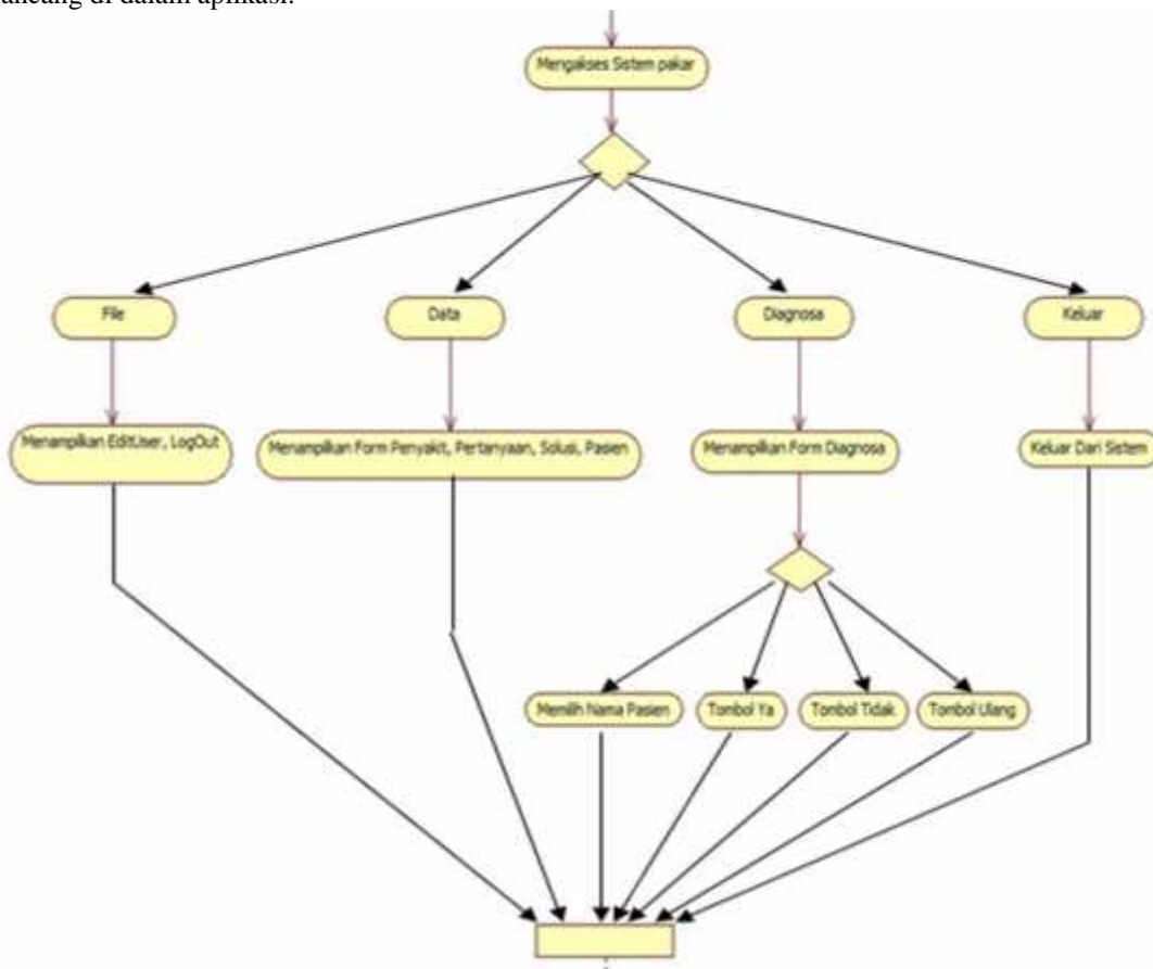
Gambar 3.4 Activity Diagram Sistem Pakar mendiagnosa Penyakit fibroid .
