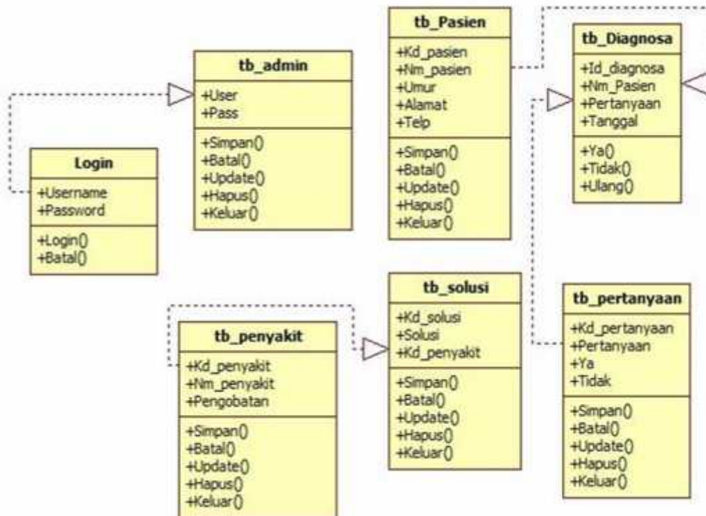
Gambar 3.2 Class Diagram Sistem Pakar mendiagnosa Penyakit fibroid.
