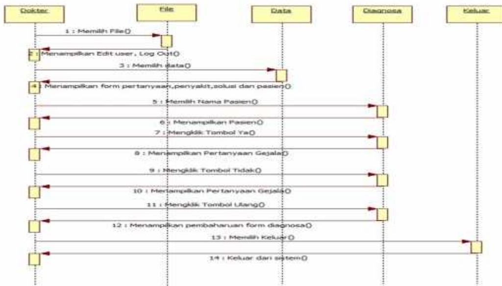
Gambar 3.3 Sequence diagram Sistem Pakar mendiagnosa Penyakit fibroid .
