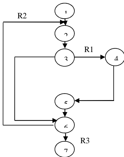
Gambar 18. Flowgraph Form Transaksi Penjualan
