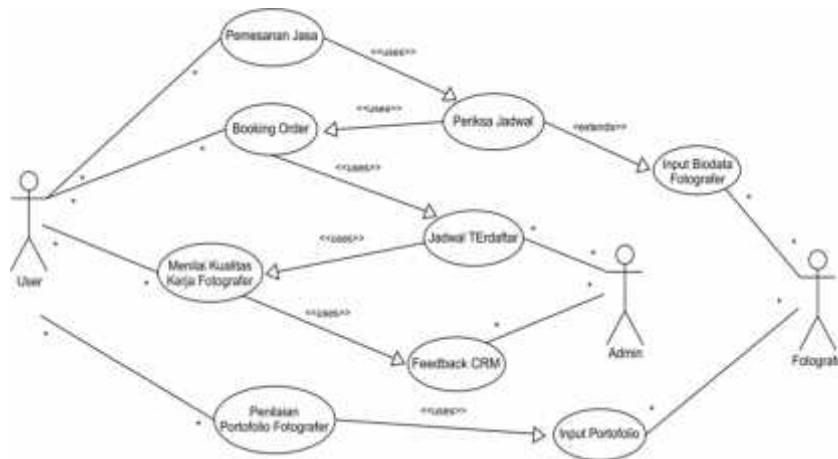
Gambar 1. Use Case Sistem Yang Diusulkan
