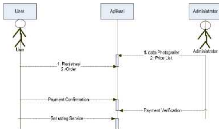
Gambar 3. Sequence Diagram Sistem yang Diusulkan
