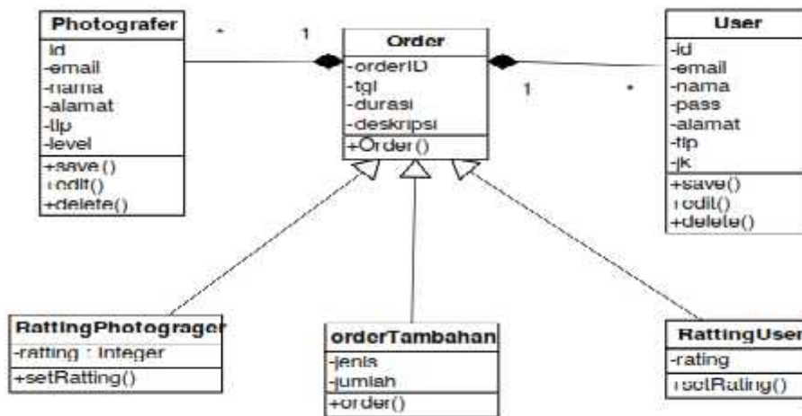
Gambar 2. Class Diagram Sistem Yang Diusulkan
