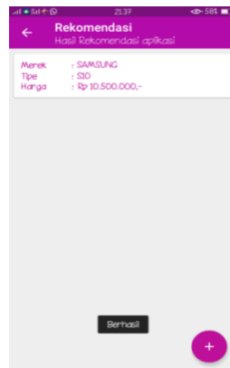
Gambar 12. Hasil Rekomendasi
