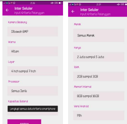
Gambar 11. Pilih Kreteria
