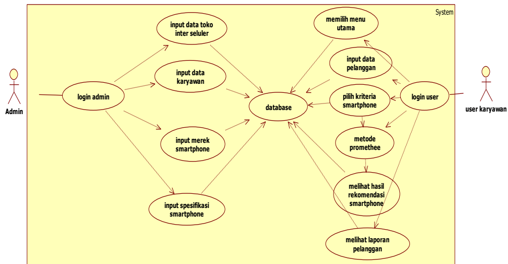
Gambar 1. Use Case Diagram Aplikasi
