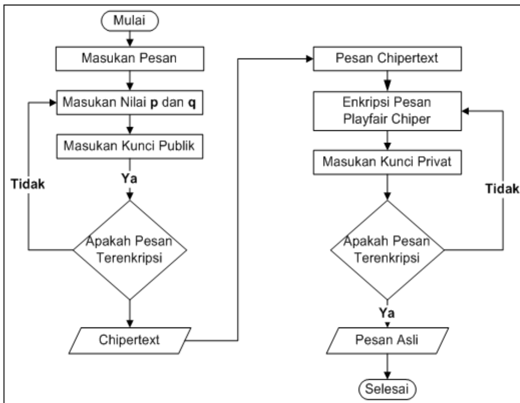
Gambar 4. flowchart Proses Plain dan Chiper Pada Algoritma RSA
