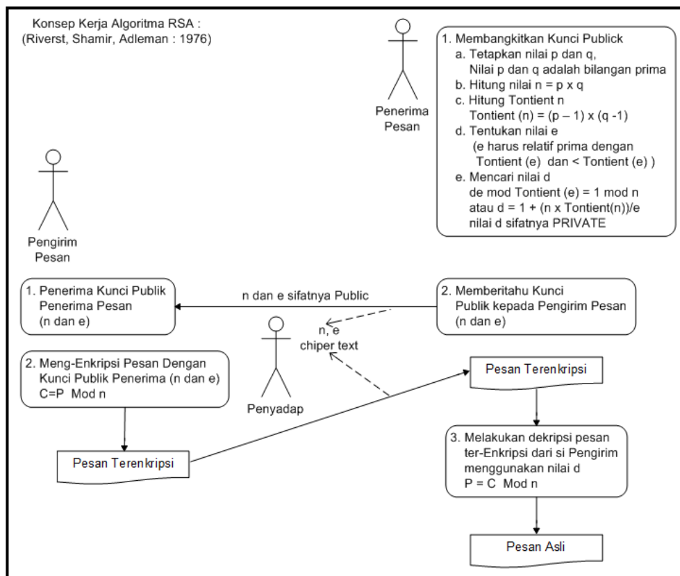
Gambar 1. Konsep Kerja Algoritma RSA
