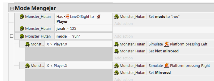
Gambar 12 Event Sheet Mode Mengejar
