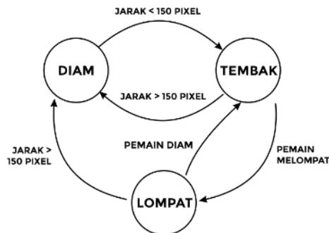
Gambar 4. Diagram Serangan Katak
