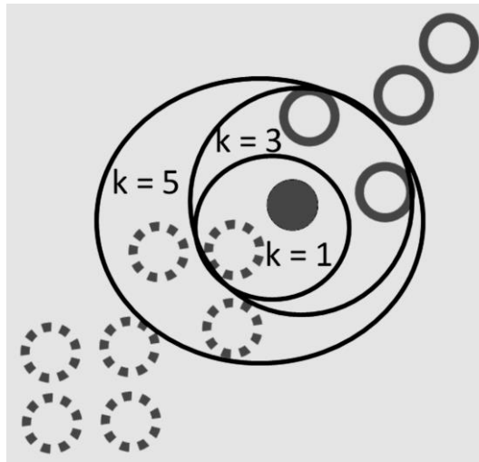
Gambar 1 : Tetangga terdekat dengan k=1, 3, dan 5 [Mayor, 2015]
