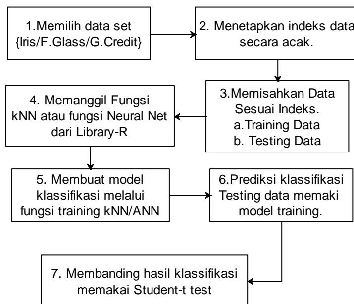
Gambar 3 : Blok Struktur Metoda Pengujian
