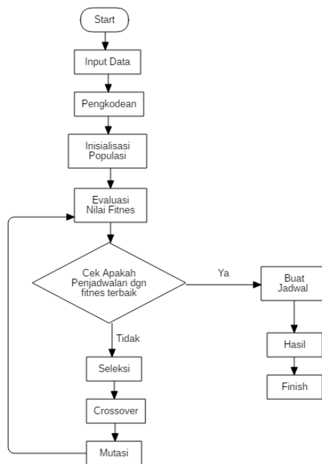
Gambar 2. Flowchart Penjadwalan dengan Metode Algoritma Genetika
