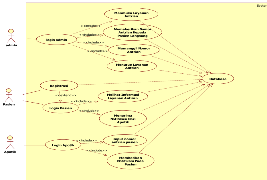
Gambar 1. Use Case Diagram Aplikasi
