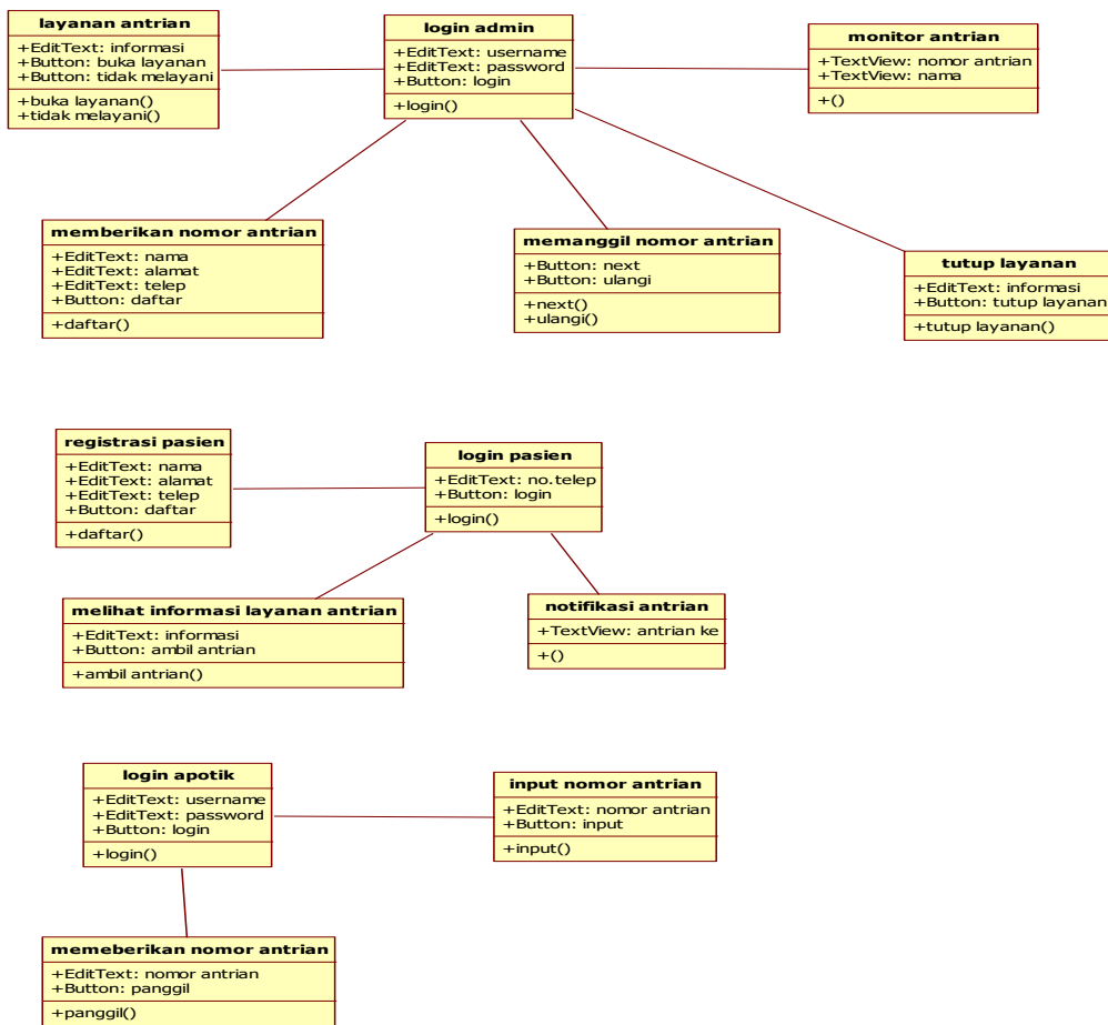
Gambar 5. Class Diagram Aplikasi
