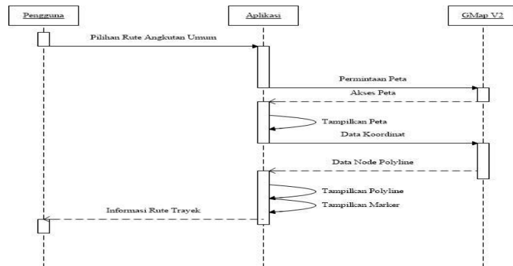
Gambar 3: Sequence Diagram Aplikasi
