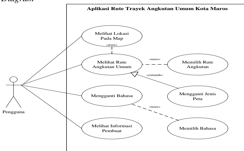
Gambar 1: Use Case Diagram Aplikasi
