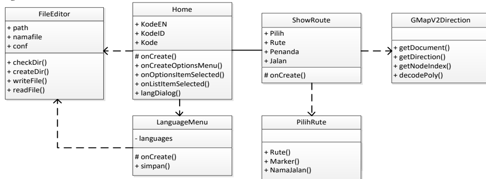
Gambar 2: Class Diagram Aplikasi
