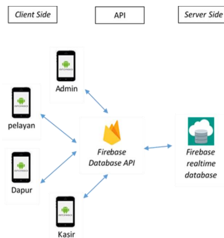
Gambar 1 Model Arsitektur
