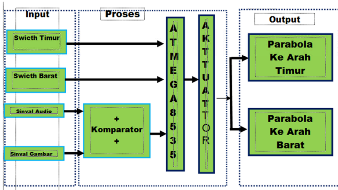
Gambar 1 Arsitektur Sistem
