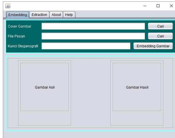
Gambar 8. Form Steganografi
