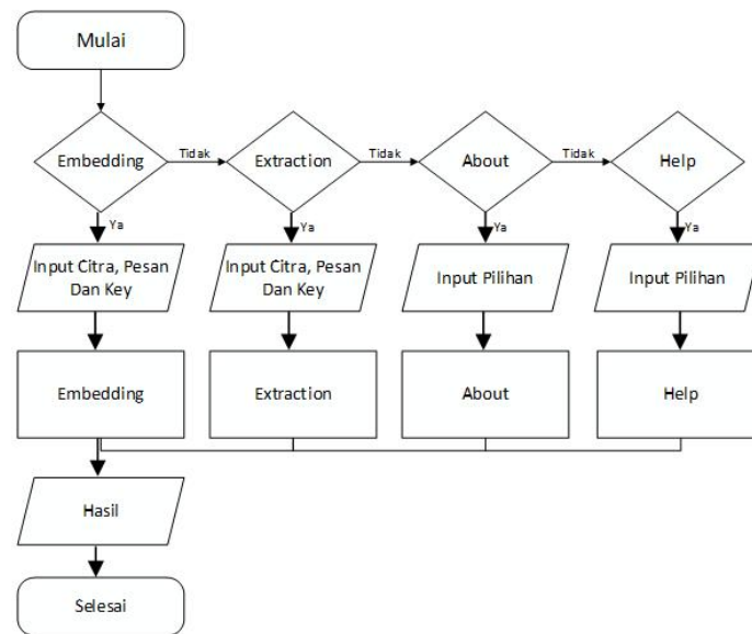
Gambar 5. Flowchart Steganografi
