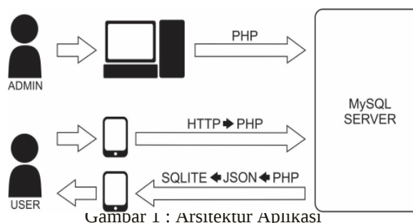
Gambar 1 : Arsitektur Aplikasi
