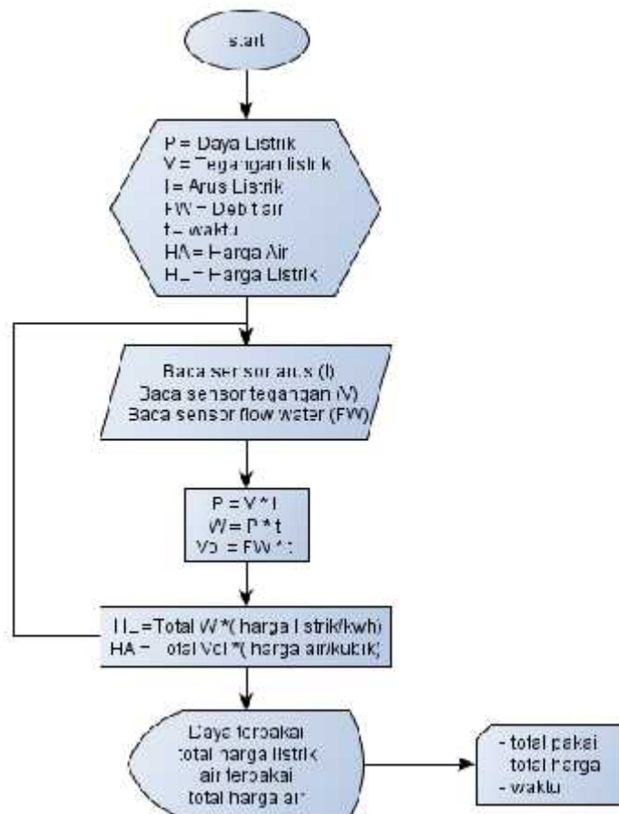
Gambar 5. Diagram Alir Utama Sistem
