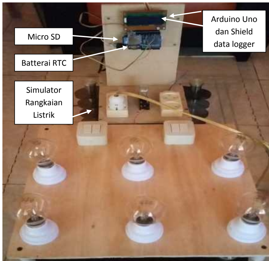
Gambar 6. Modul Arduino dan Simulator Rangkaian Listrik
