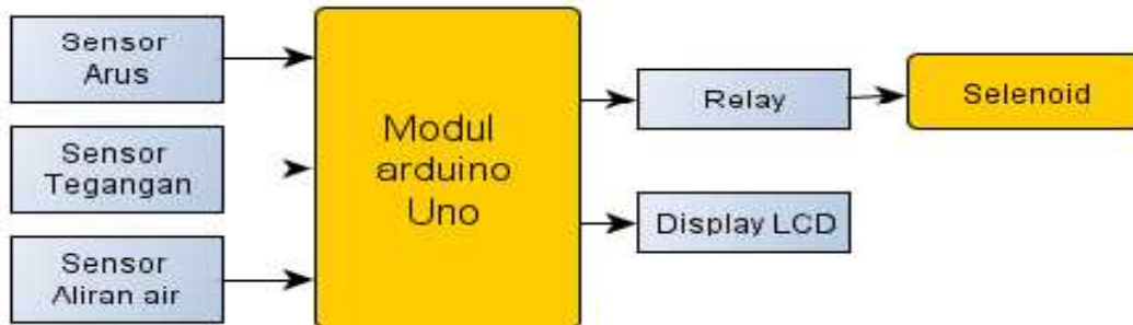
Gambar 4. Diagram Blok Rangkaian
