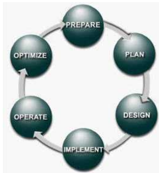
Gambar 2. Metode PPDIOO
