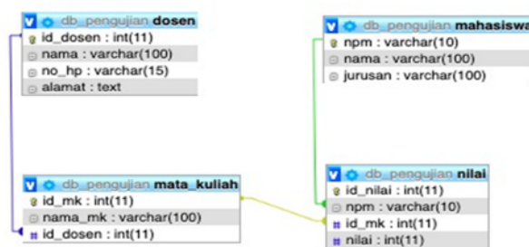
Gambar 3. Relasi Tabel
