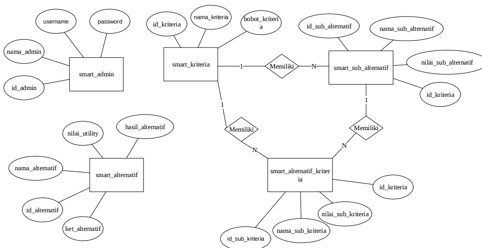
Gambar 2. ER D Diagram
