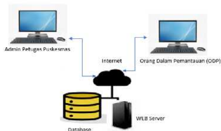
Gambar 4. Arsitektur SI Pantau ODP
