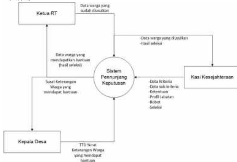
Gambar 3. Diagram Konteks
