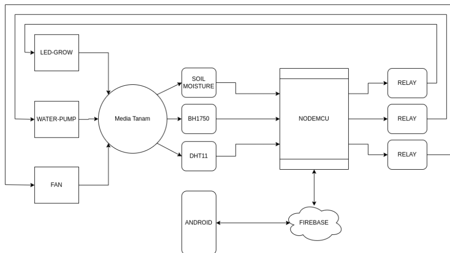
Gambar 2 Blok diagram perancangan perangkat keras
