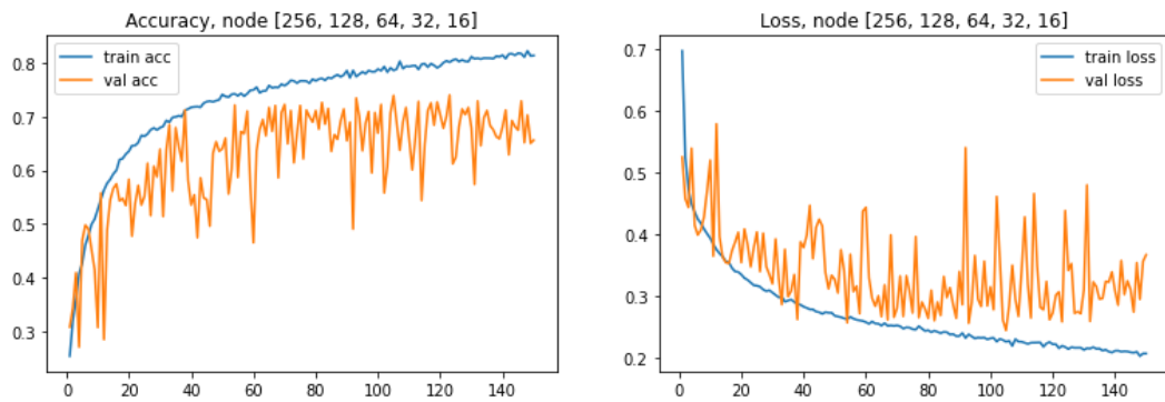
Gambar 4.3 Output skenario ke-3 Adam 90% Training dan 10% Testing
