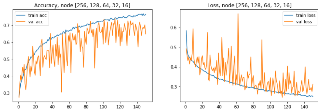
Gambar 4.4 Output skenario ke-1 SGD 80% Training dan 20% Testing
